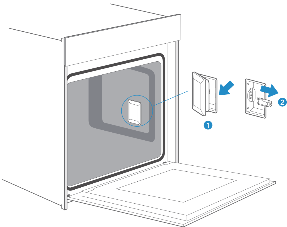
Bočna žarulja
