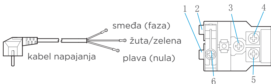
priključna kutija
